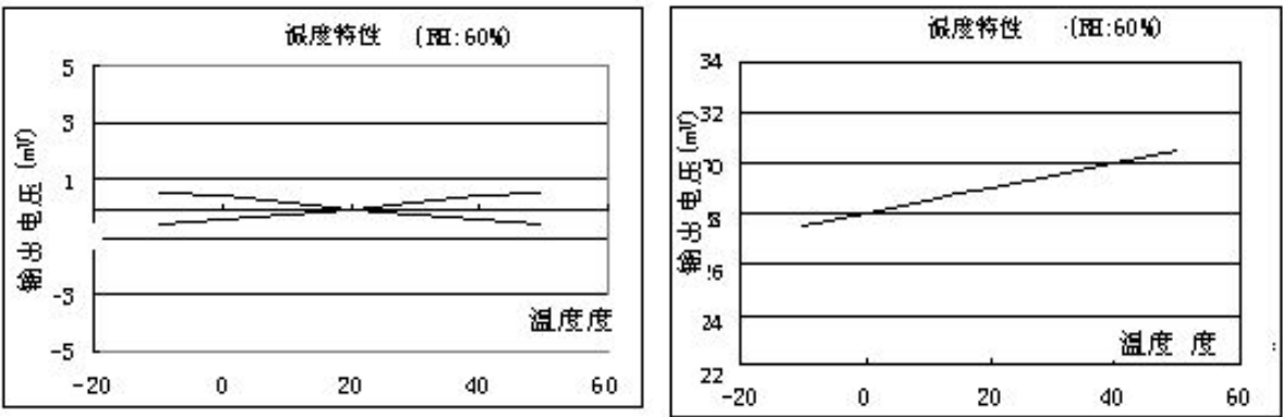
图 5 ： 零点温度特性曲线
