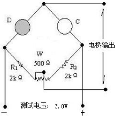
图 2：基本测试电路
